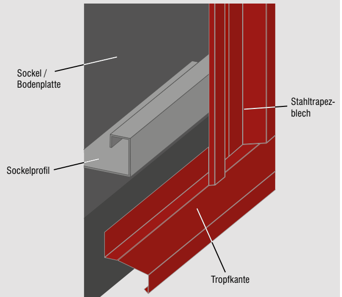
Wandverkleidung mit Stahltrapezblechen
